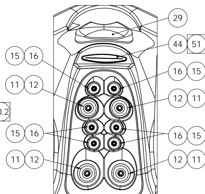
B (1 : 10)
